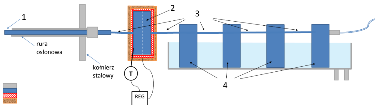
Rys. 1 Schemat linii próbkowania gazu. 1: sonda; 2: obudowa filtra; 3: elementy łączące; 4: płuczki.
